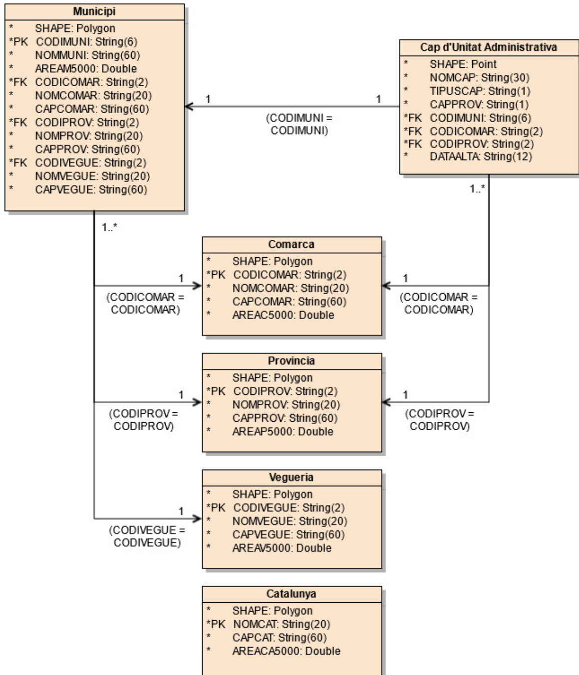
Figura 2. Esquema d'implementació del model de dades de Divisions administratives v2.0 en format SHP
