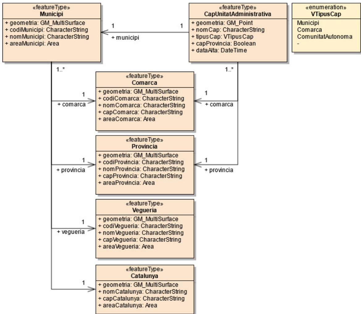
Figura 1. Esquema conceptual del model de dades de Divisions administratives v2.0
