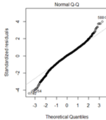
Imatge 2. Distribució dels residus en les cues dels diagrames Q-Q plot
