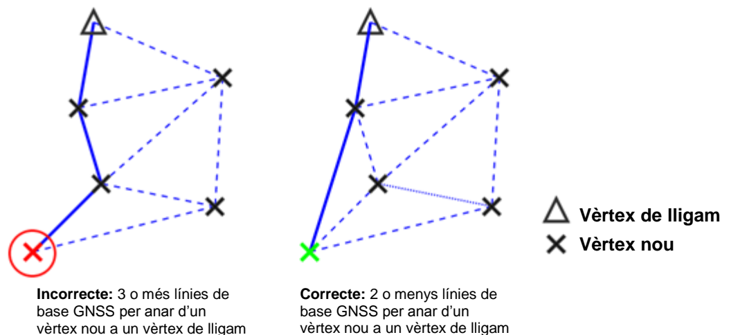
Figura 2 Requeriment per a la distribució de bases GNSS
