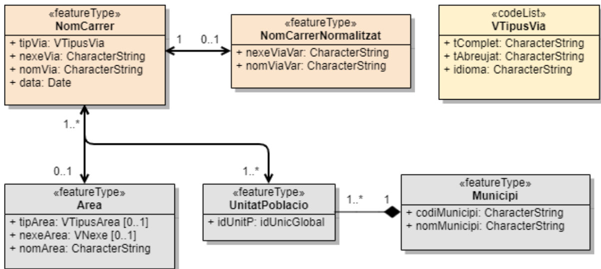
Figura 1: Esquema conceptual del model de dades dels noms de carrer v2.0
