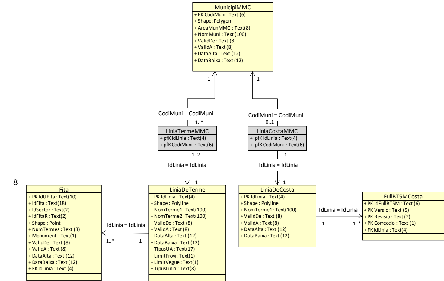
Figura 1 - Diagrama de classes UML del model de dades físic del Mapa municipal de Catalunya 1:5 000 (MMC-5M) v1.0 per al format Shapefile.
